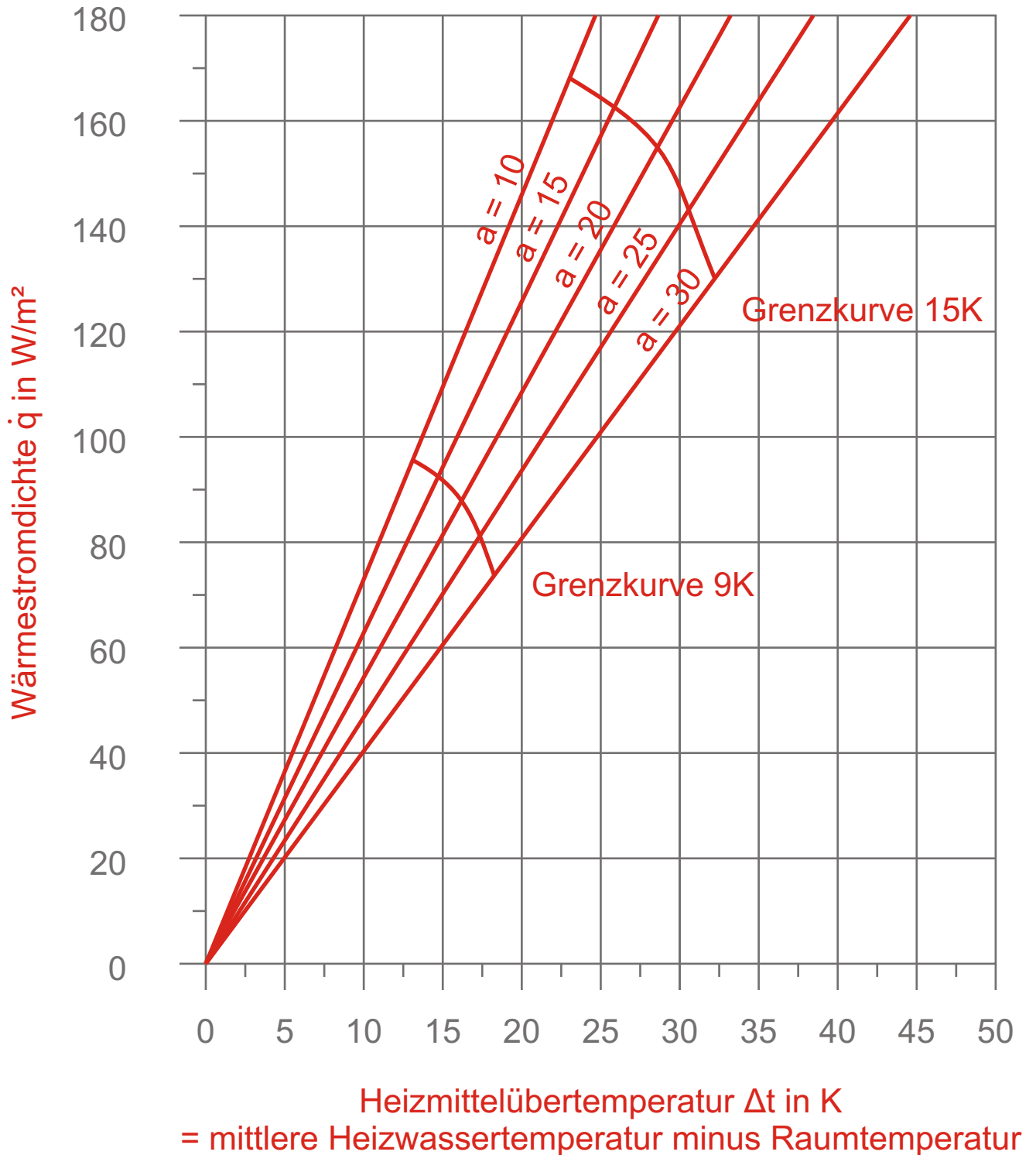
Diagramm 5 Oberbelag R_{\lambda} = 0,0 \text{ m}^2\text{K/W} Fliesen und Steinbeläge PVC und Linoleum bis 3 mm geklebt
