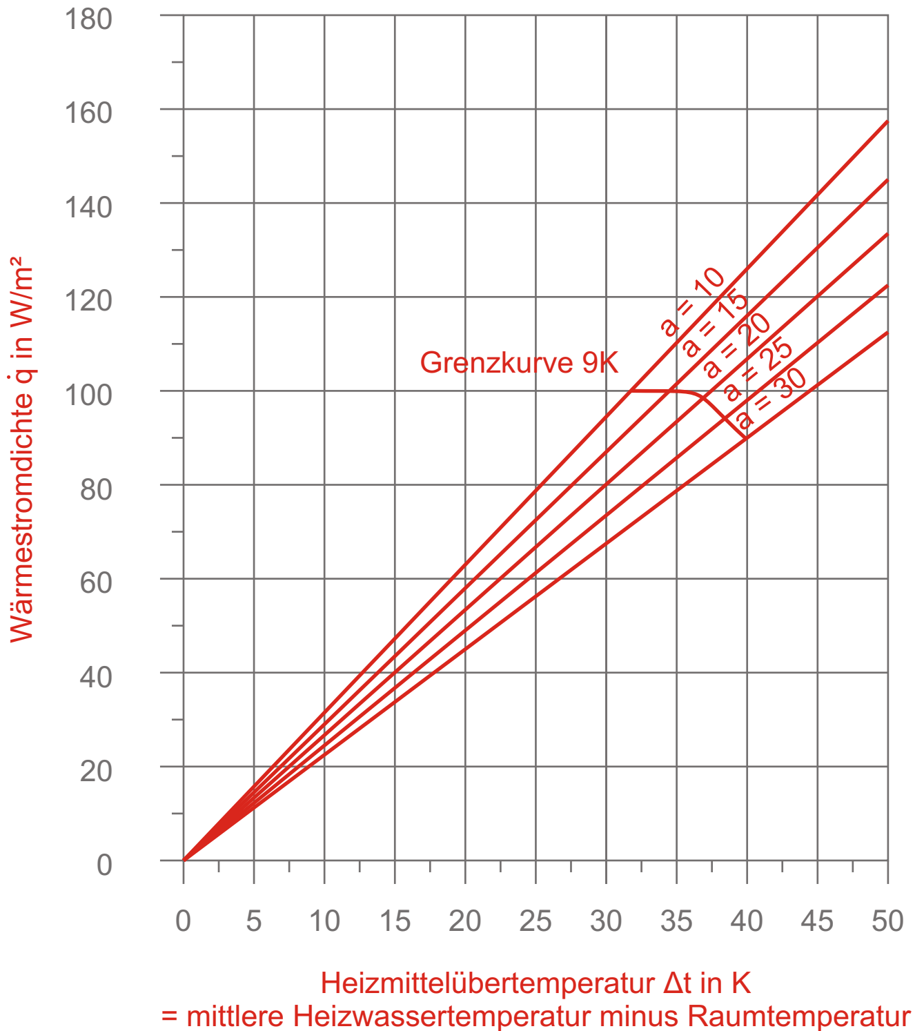
Diagramm 4 Oberbelag R_{\lambda} = 0,15 \text{ m}^2\text{K/W} Teppich, Parkett 22 mm
