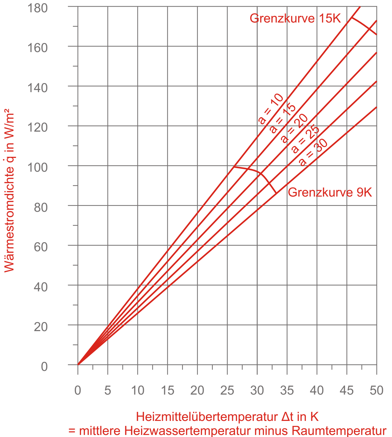
Diagramm 3 Oberbelag R_{\lambda} = 0,10 \text{ m}^2\text{K/W} Teppich, Parkett 15 mm
