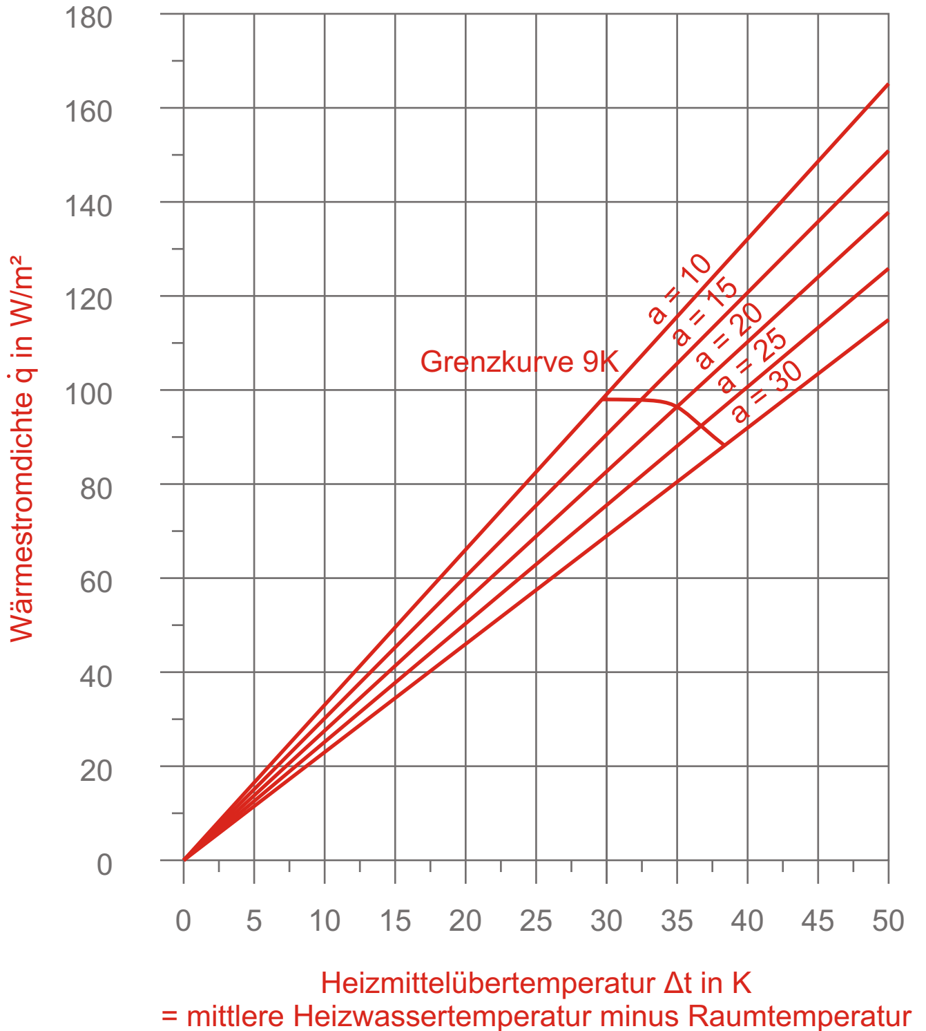
Diagramm 8 Oberbelag R_{\lambda} = 0,15 \text{ m}^2\text{K/W} Teppich, Parkett 22 mm
